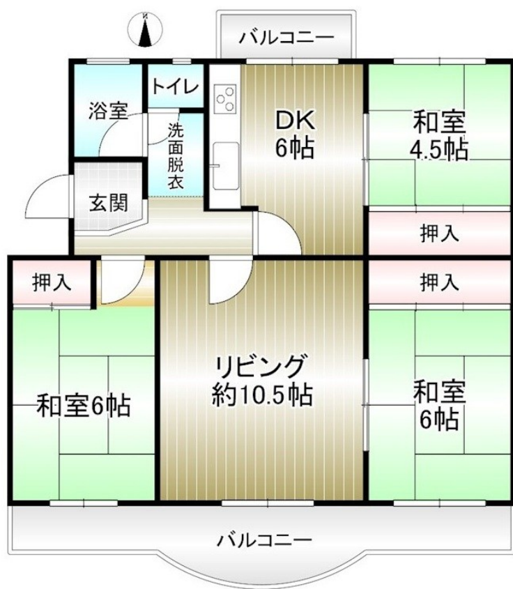
【間取り図】
